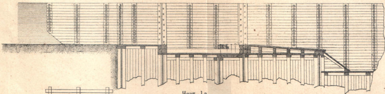
Черт. 1а. Планъ верховой шлюзной части.
