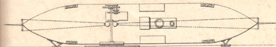
Фасадъ.
