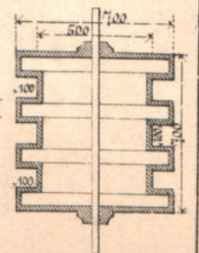
Черт. 6г. Разрѣзъ по NO (6в.)
