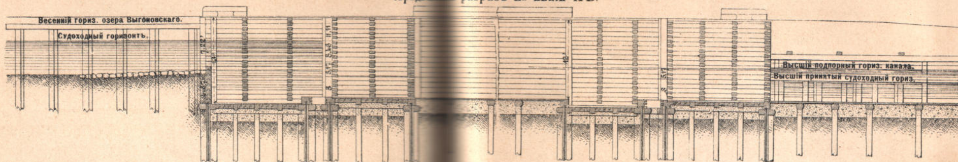
Черт. 1. Продольный разрезъ по линіи АВ.
