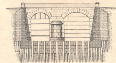
Поперечный разръзъ по линіи LM.
