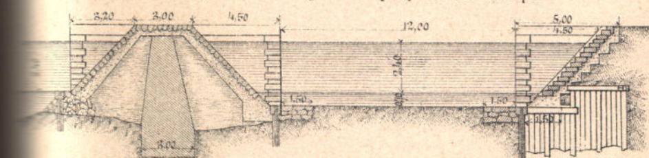
Черт. 6в. Прод. разръзъ верхней шлюзн. части
