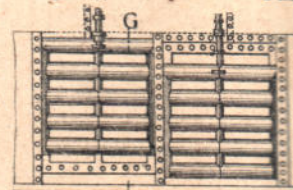
Фасадъ щитовъ.
