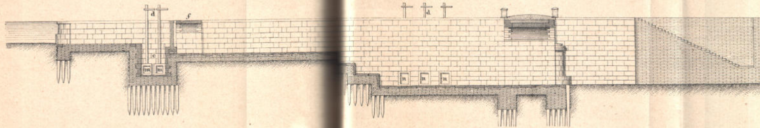
Продольный разръзъ по линіи СД.
