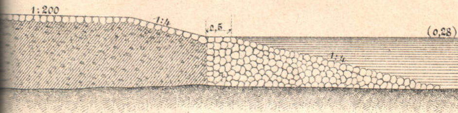
Черт. 5. Поперечный разръзъ.
