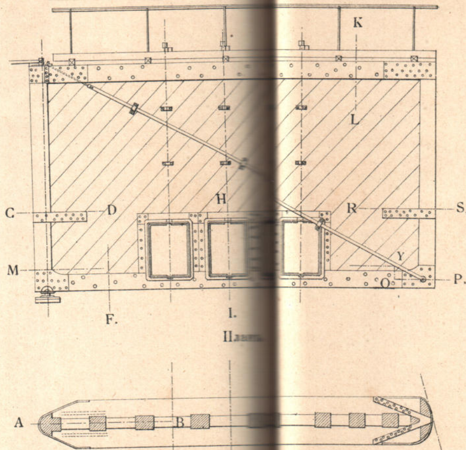
Разрѣзъ по HI.
