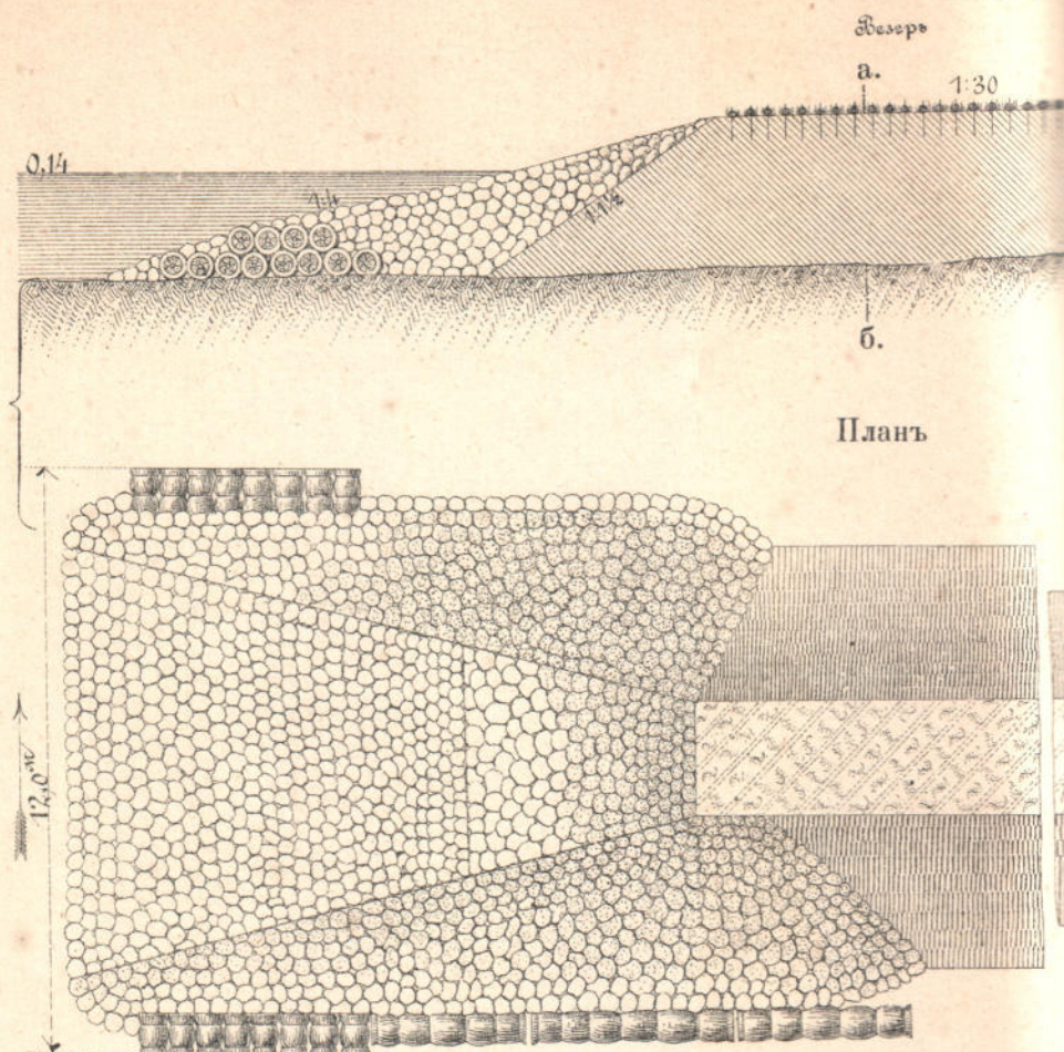
Черт. 1. Продольный разръзъ
