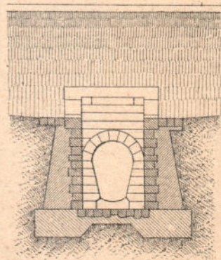
Поперечный разръзъ по колодцу.
