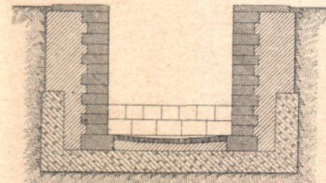
Черт. 4. Разрезъ по С D.
