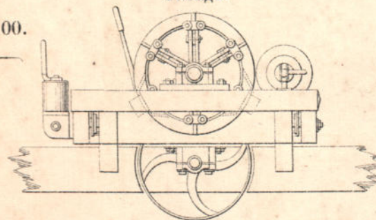
Черт. 103. Фасадъ.
