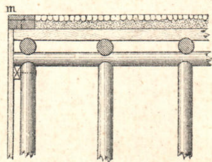
Черт. 5. Разрѣзъ.
