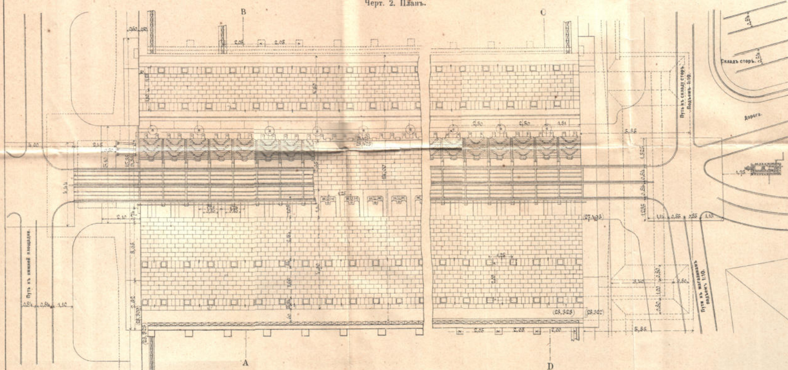
Черт. 2. Планъ.
