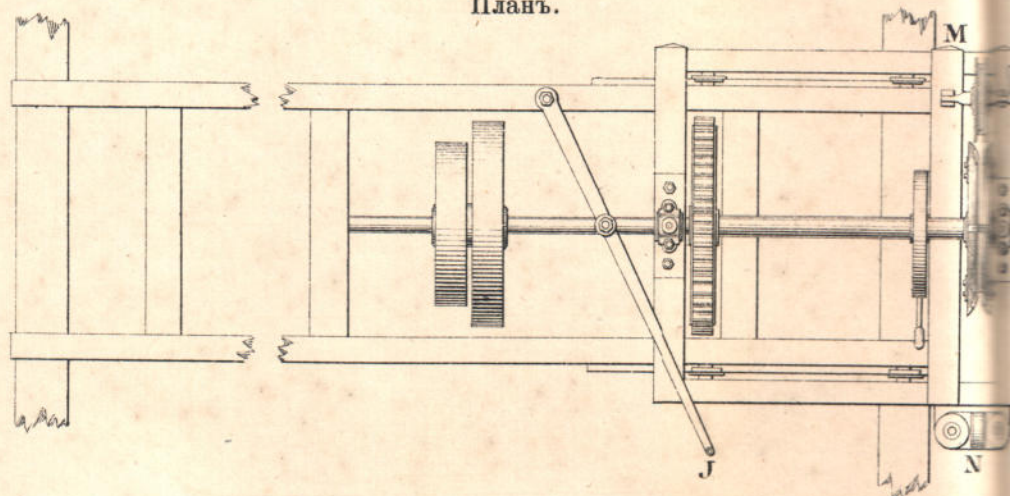
Планъ.
