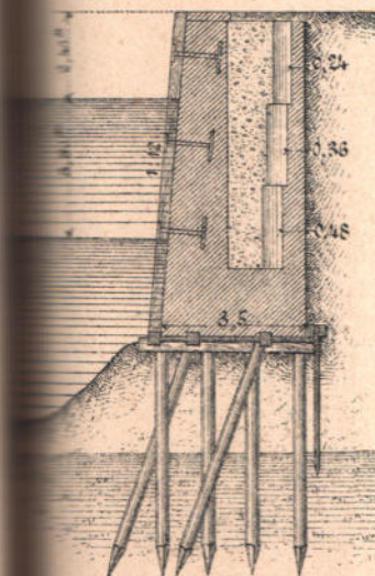
Черт. 8. Разрѣзъ.
