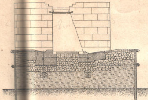
Разрѣзъ по СD.
