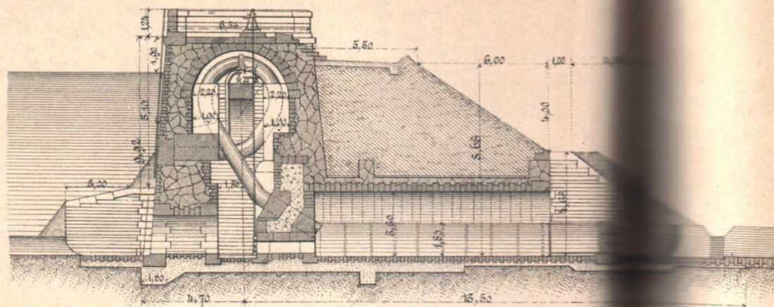
Черт. 1. Разрѣзъ по оси
