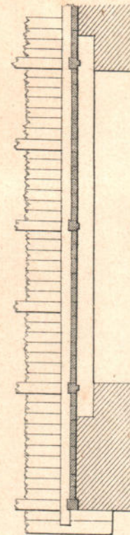
Черт. 2 д. Разрѣзъ по ЕФ.
