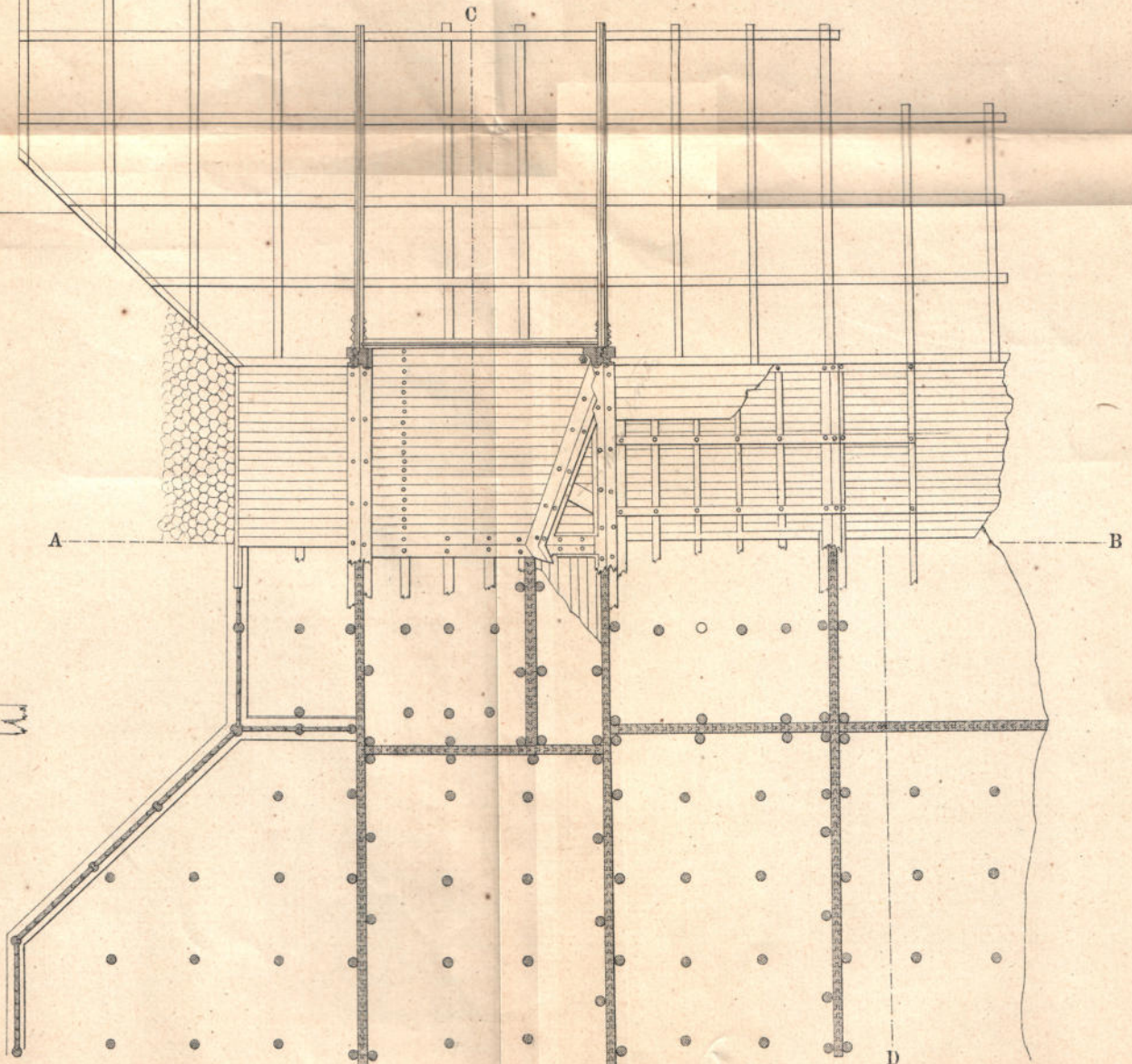
Черт. 1а. Планъ верховой шлюзной части.
