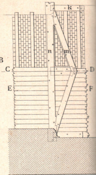
Черт. 2 г. Разрѣзъ по СД.
