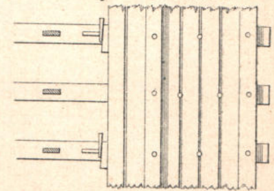
Черт. 4 б. Планъ.
