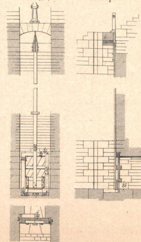
Фасадъ, Черт. 6. Разрѣзъ.
