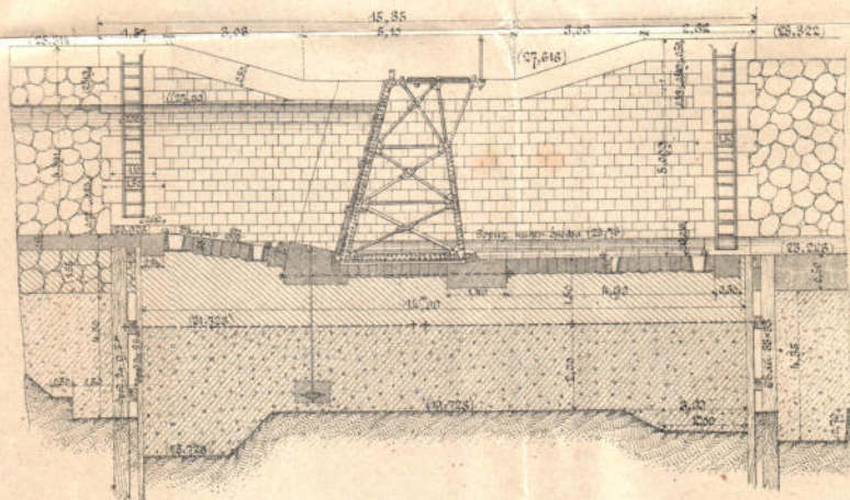
Черт. 4. Поперечный разръзъ по CD.
