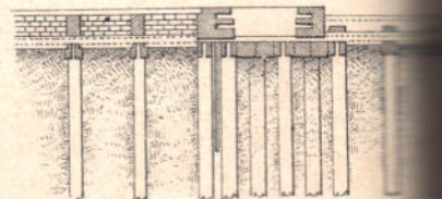
Черт. 2 г. Разрѣзъ по СД.
