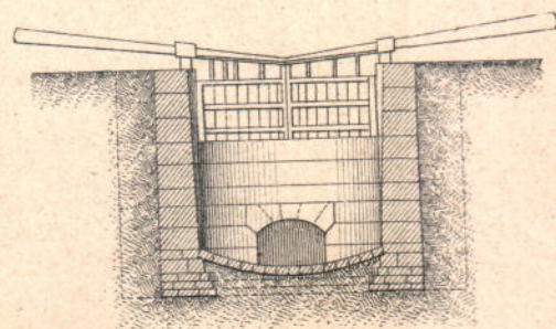
Черт. 1 в. Разрѣзъ по С D.
