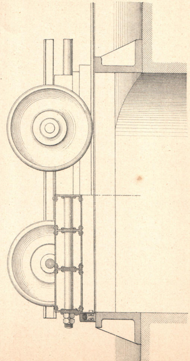
Черт. 3. Разрѣзъ и боковой видъ по abcd. (черт. 2).
