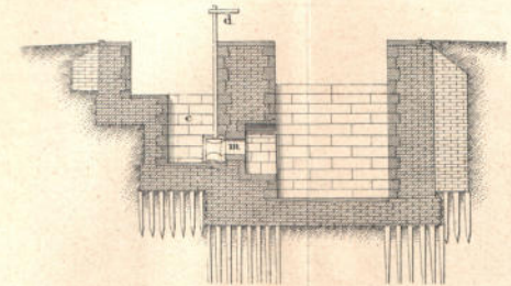
Поперечный разръзъ по линіи СН.
