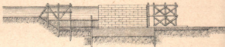
Продольный разръзъ верхней головы шлюза по оси камеры.
