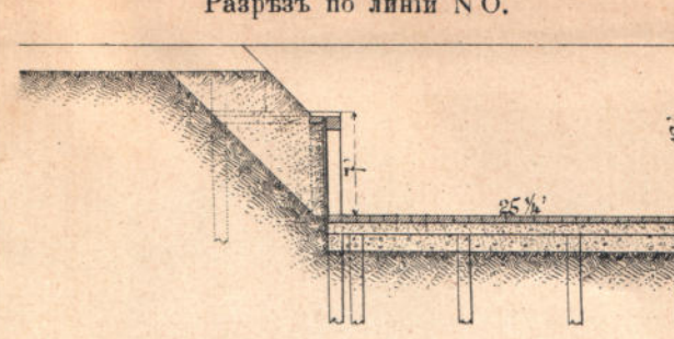
Разрезъ по линіи NO.
