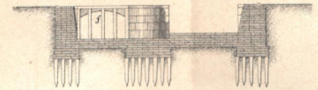
Поперечный разръзъ по линіи ЕФ.
