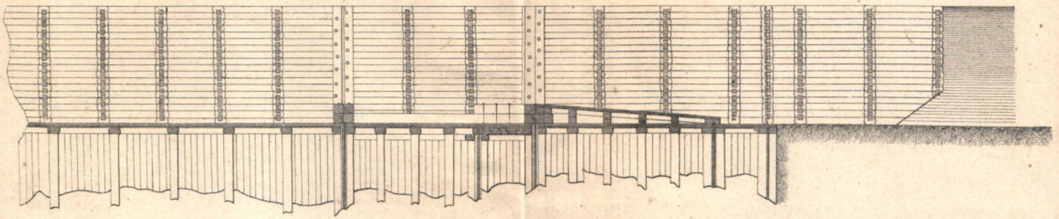
Черт. 1б. Верховая шлюзная часть. Разрѣзъ по А В.
