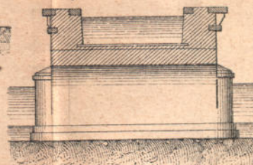
Поперечный разрѣзь.
