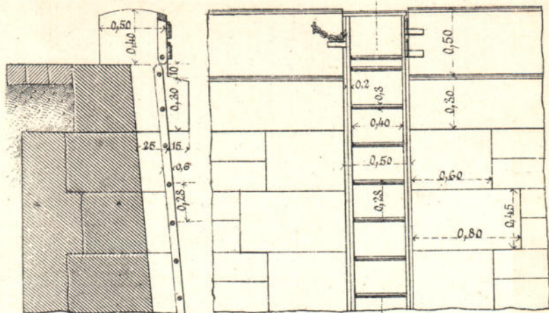
Черт. 2. Фасадъ.
