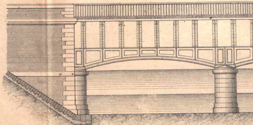
Черт. 3а. Фасадъ.
