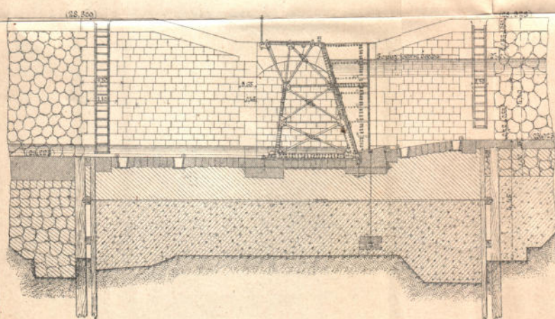
Черт. 3. Поперечный разрезъ по АВ.
