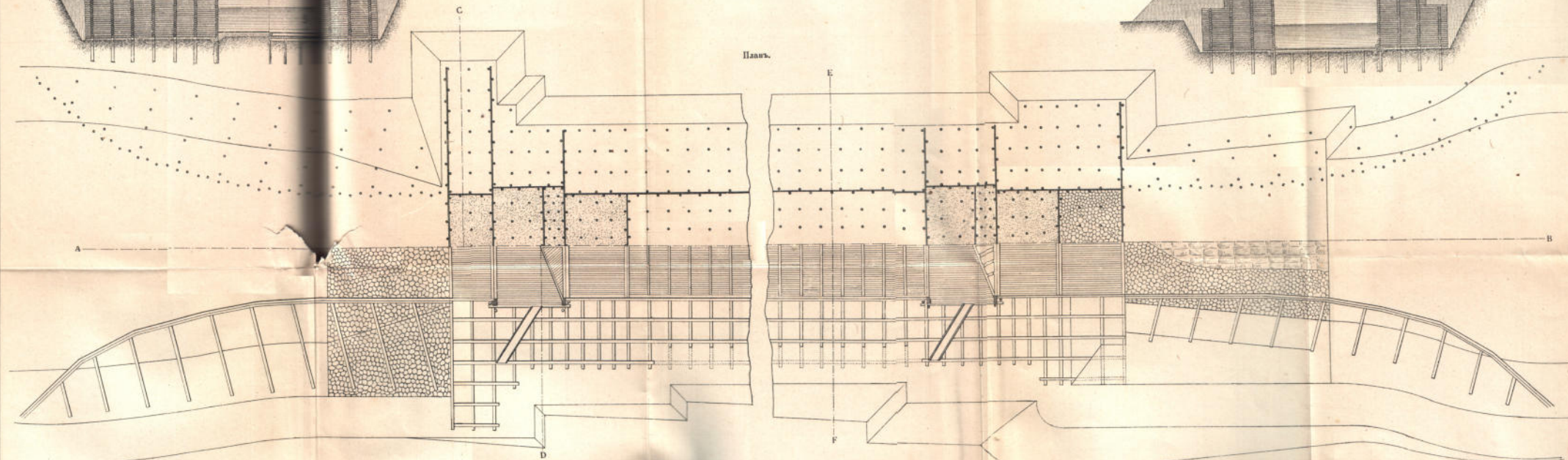
22,00 Разрѣзъ по С D.
