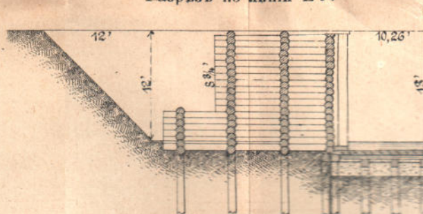
Разрезъ по линіи EF.
