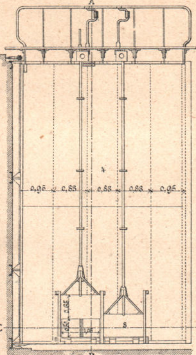
Черт. 2 в. Разрѣзъ по СД.
