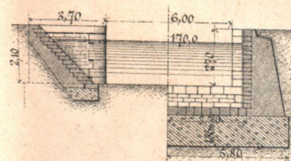
Черт. 2б. Четр. 2в. Разрѣзъ по EF. Разрѣзъ по GH.
