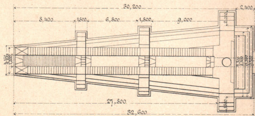
Черт. 4. Планъ.
