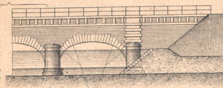
Черт. 4б. Фасадъ.
