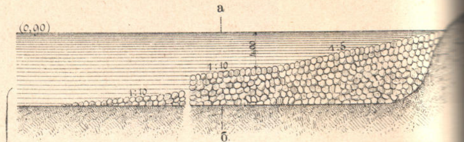
Разрѣзъ по а б.
