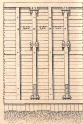
Фасадъ.
