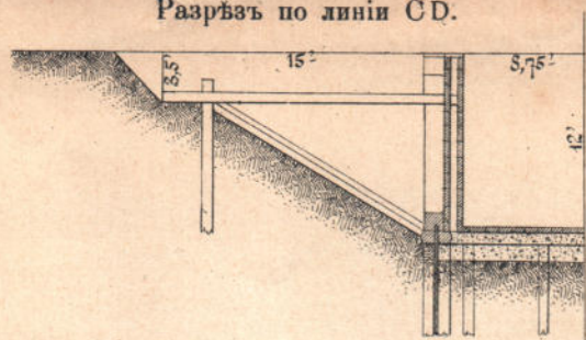
Разрезъ по линіи CD.
