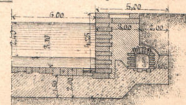
Черт. 6д. Разръзъ по АВ.
