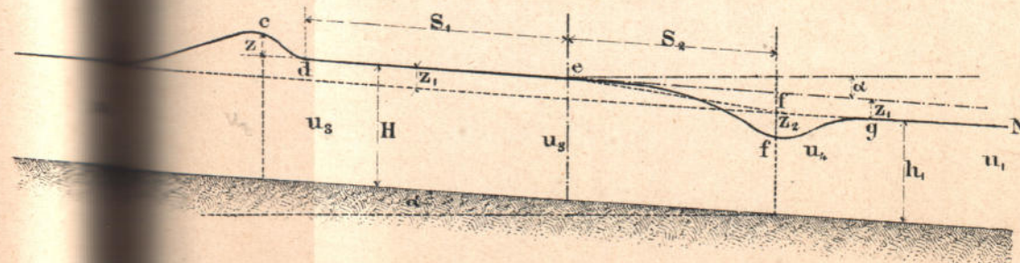
Черт. 8б. Продольная профиль по MN
