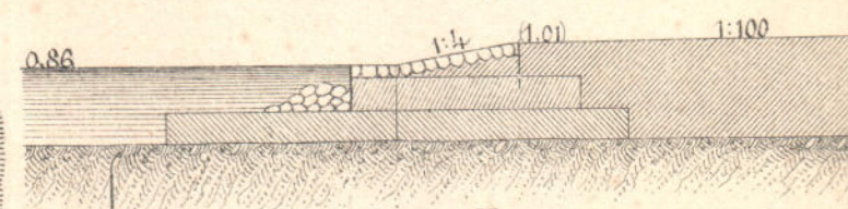
Черт. 4. Продольный разръзъ.
