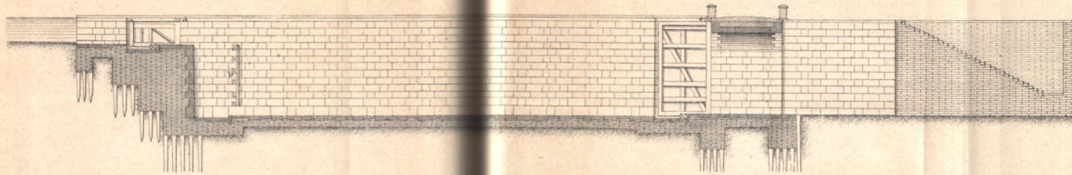
Продольный разръзъ по линіи СД.
