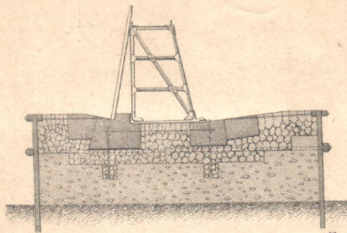
Разрѣзъ по АВ.
