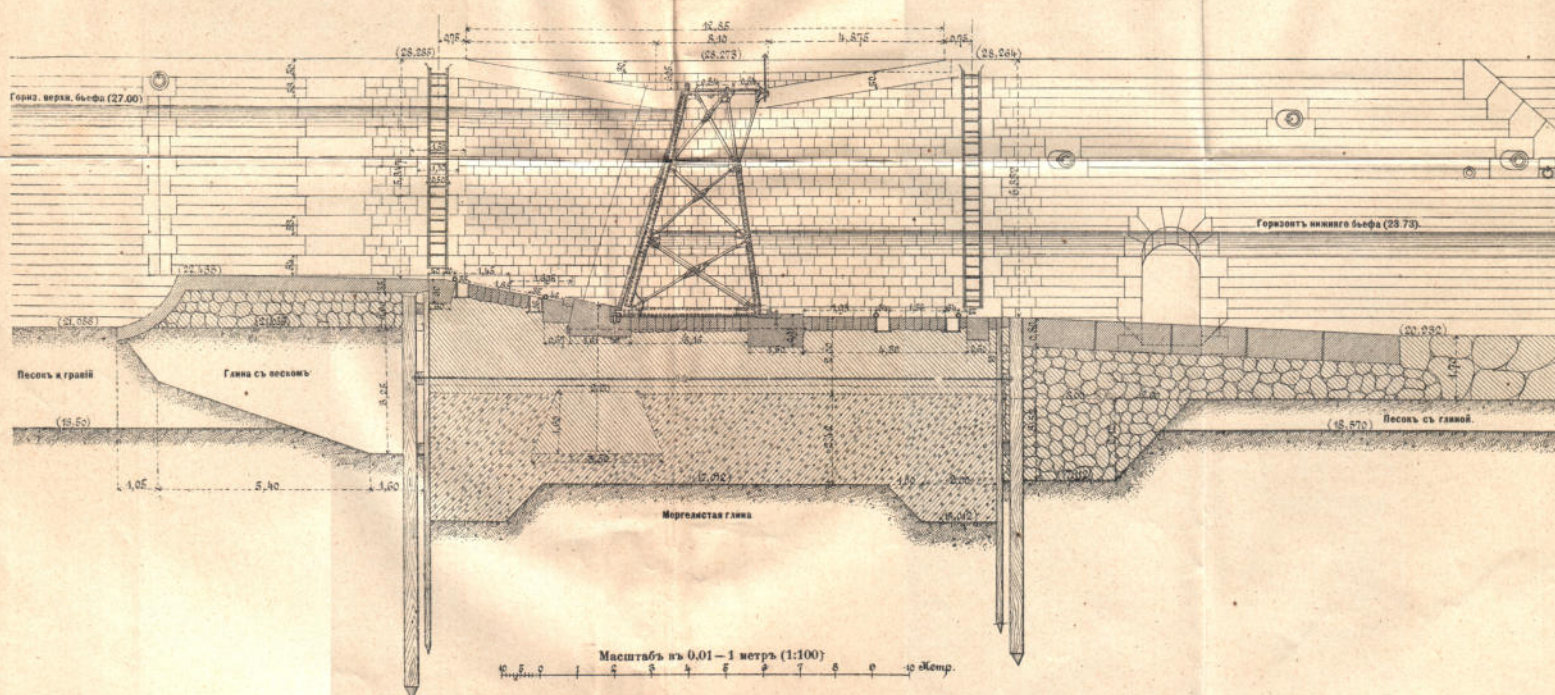
Черт. 3. Поперечный разрезъ
