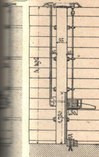
Разрѣзъ.
