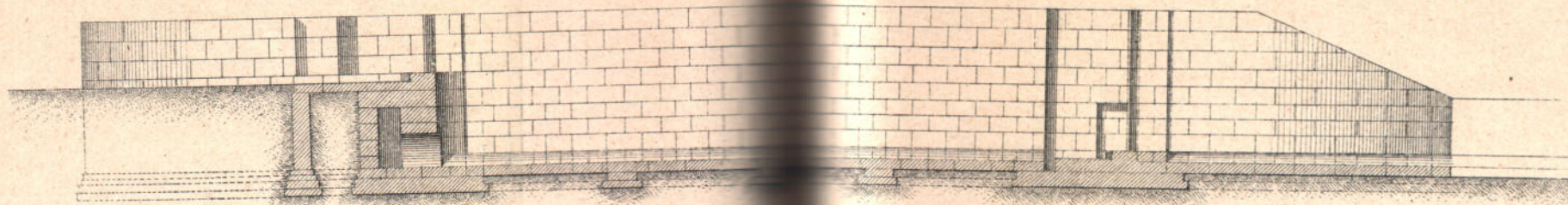
Черт. 1а. Продольный разрезъ.
