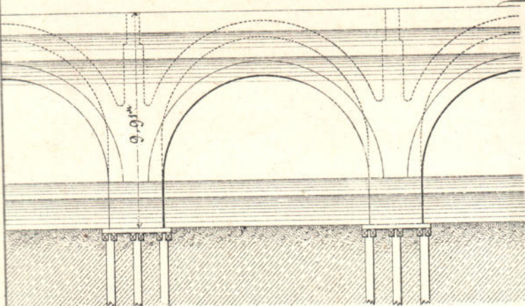
Фасадъ.
