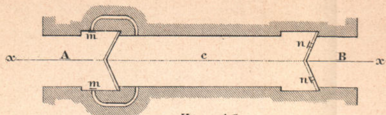
Черт. 1 б. Схема разреза по ослхх
