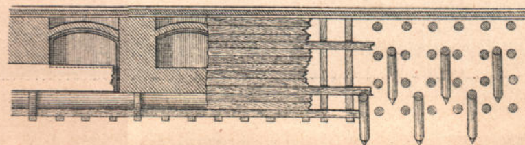
Черт. 10. Планъ.
