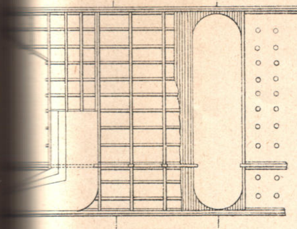
Черт. 2. Планъ.
