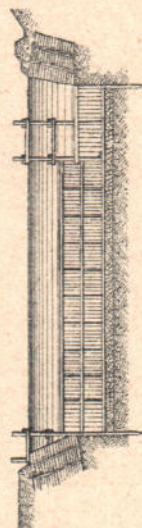
Поперечный разръзъ верхней головы шлюза по стѣнкѣ паденія и ниже ея.
