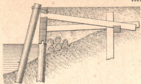
Черт. 3. Разрѣзъ.
