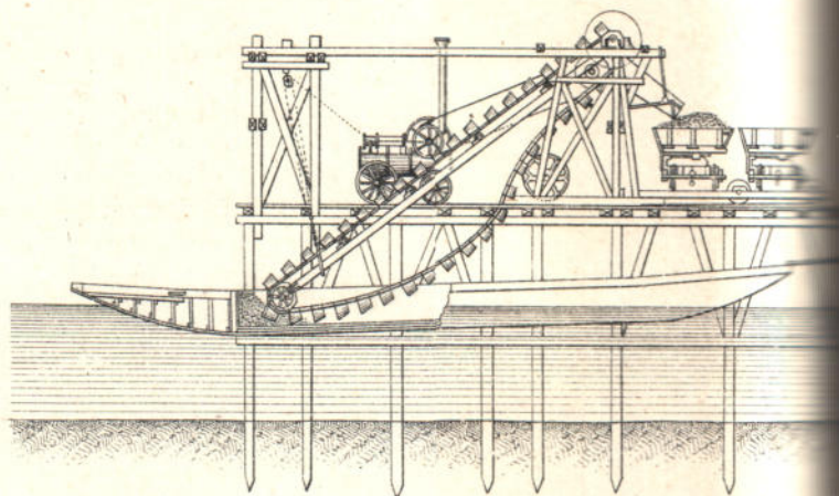
Черт. 2. Фасадъ.
