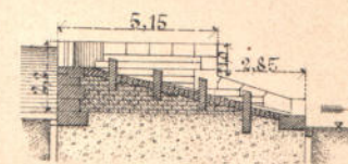
Черт. 4 б Разрѣзъ а б.
