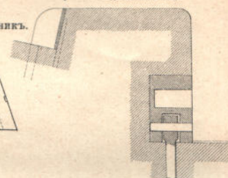
Разрѣзъ подфермнаго камня по оси верхняго подшипника АВ.
