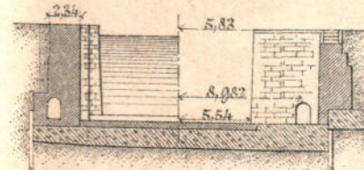
Черт. 2б. Четр. 2в. Разрѣзъ по EF. Разрѣзъ по GH.
