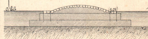
Разръзъ по а б.
