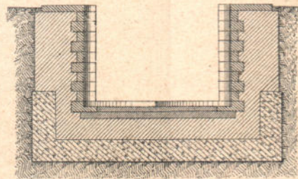
Черт. 3. Разрезъ по А В.
