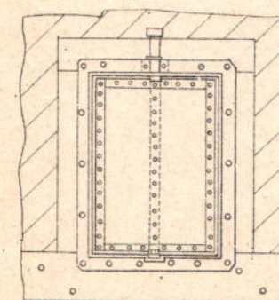
Щитъ.
