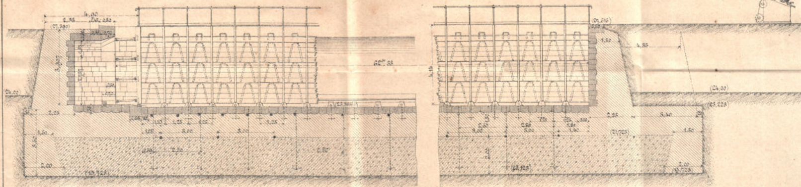
Черт. 1. Продольный разрезъ. Видъ со стороны нижняго бьефа.
