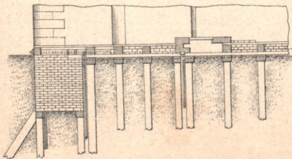
Черт. 1 б. Разрѣзъ по АВ.
