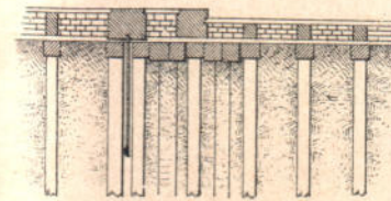
Черт. 2 д. Разрѣзъ по ЕФ.
