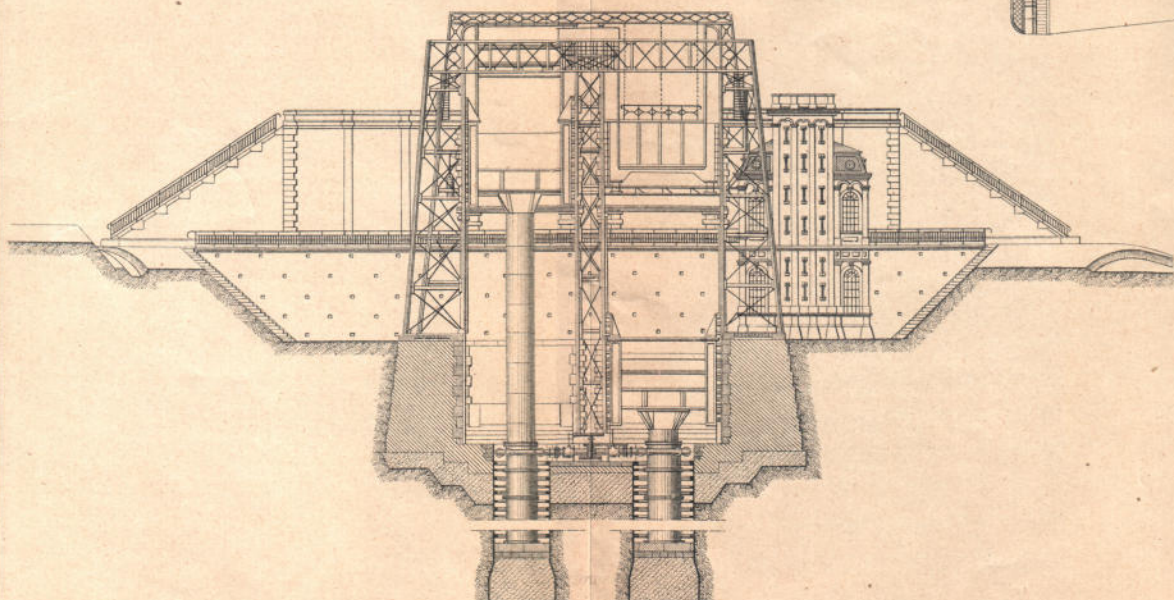
Поперечный разръзъ.
