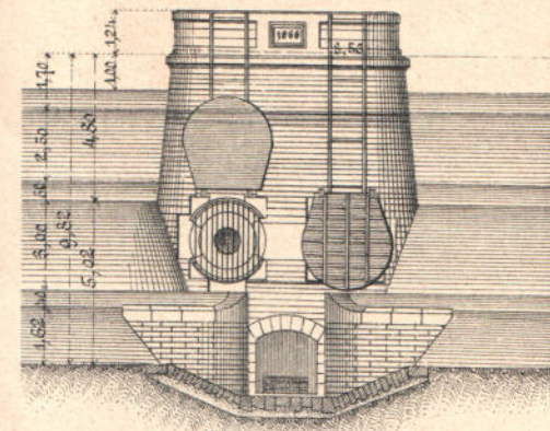
Черт. 3. Фасадъ башни.
