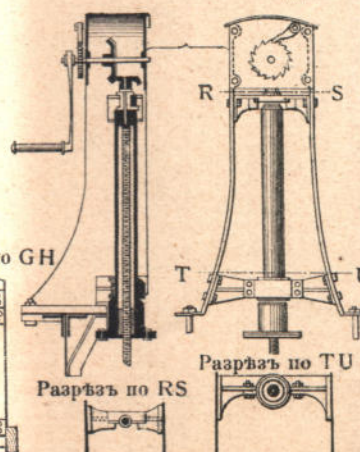
Черт. 4. Домкратъ для подъема щита.
