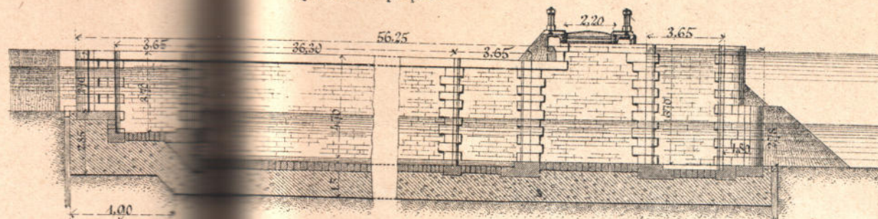
Черт. 1в. Разрѣзъ по АВ. Фасадъ низ...
