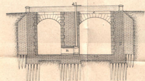
Поперечный разръзъ по линіи LM.
