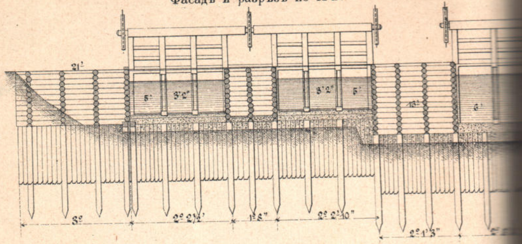
Фасадъ и разръзъ по А В.
