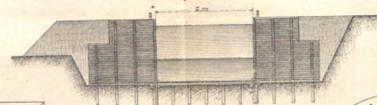
Разрѣзъ по E F.
