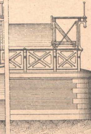
Поперечный разрѣзь.
